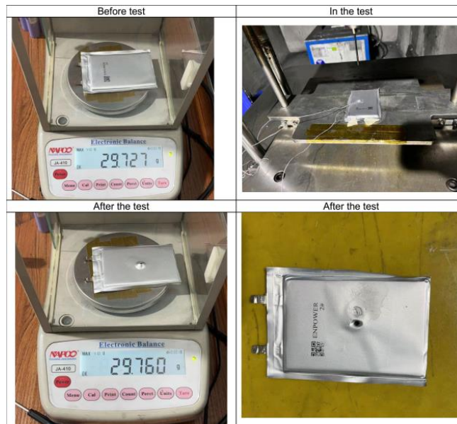
第三方测试机构报告示图（针刺前后电芯状态）
